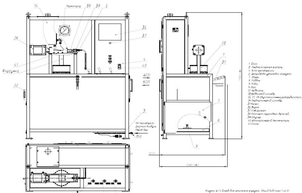
Рисунок 4.1 – Стенд для испытания форсунок. Общий вид (лицевая сторона)
