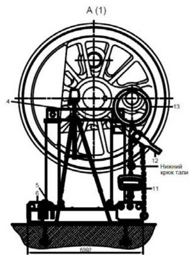
4 - нож; 5 - тяжелая скоба; 6 - пластина; 11 - кантовые весы; 12 - таль; 13 - ядро
