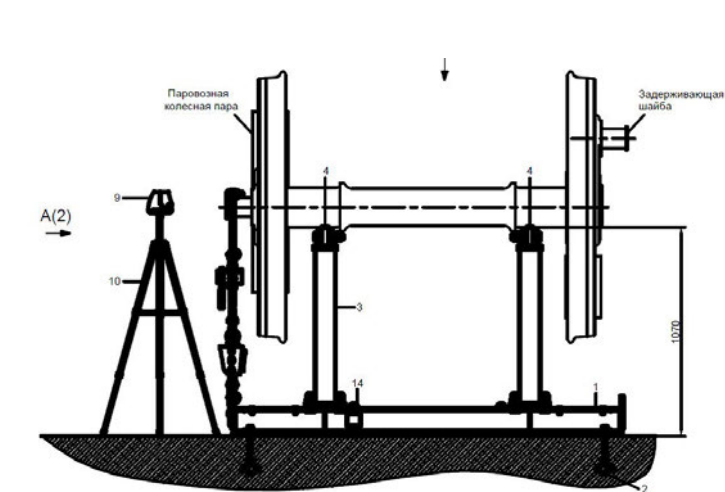
Рисунок А.1 - Общий вид стенда при балансировке (лист 1 из 3)
